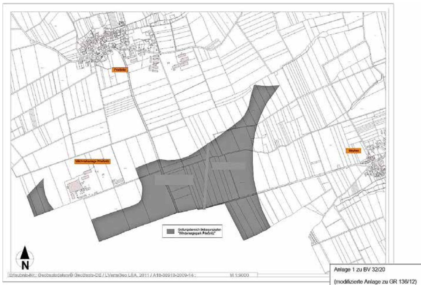
Anlage 1: Räumlicher Geltungsbereich Bebauungsplan „Windenergiepark Prießnitz“ der Stadt Naumburg (Saale)
